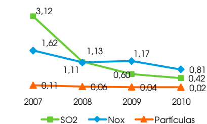
Emissões Específicas parque térmico NO x , SO 2 e partículas (g/kWh)
