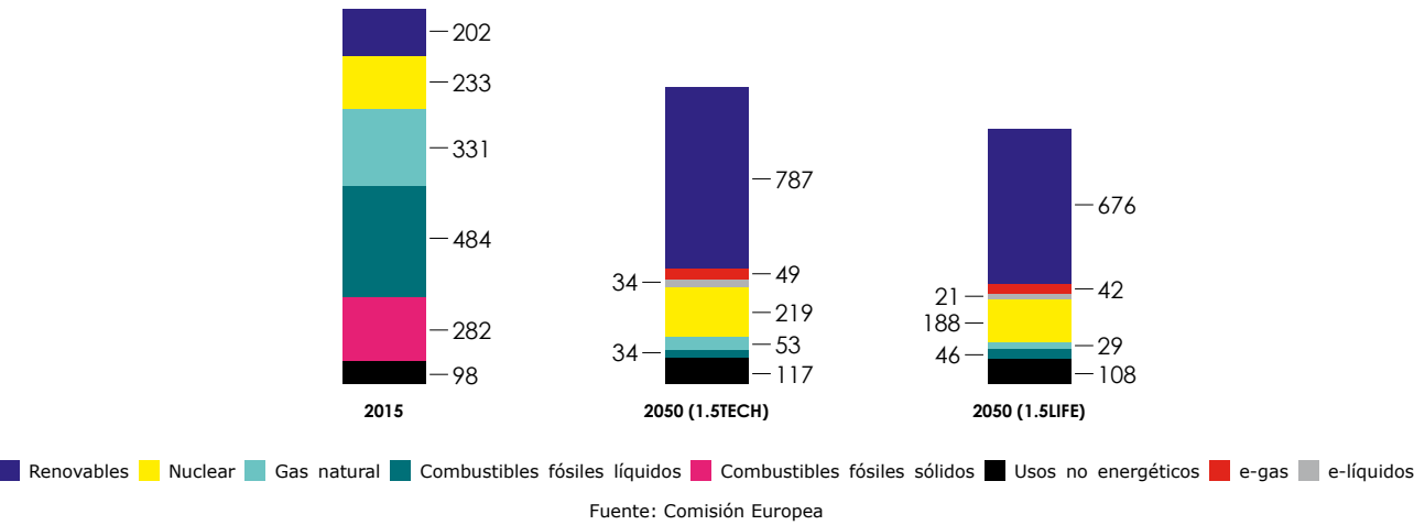
ENERGÍA PRIMARIA EN LA UE (Mtep)
