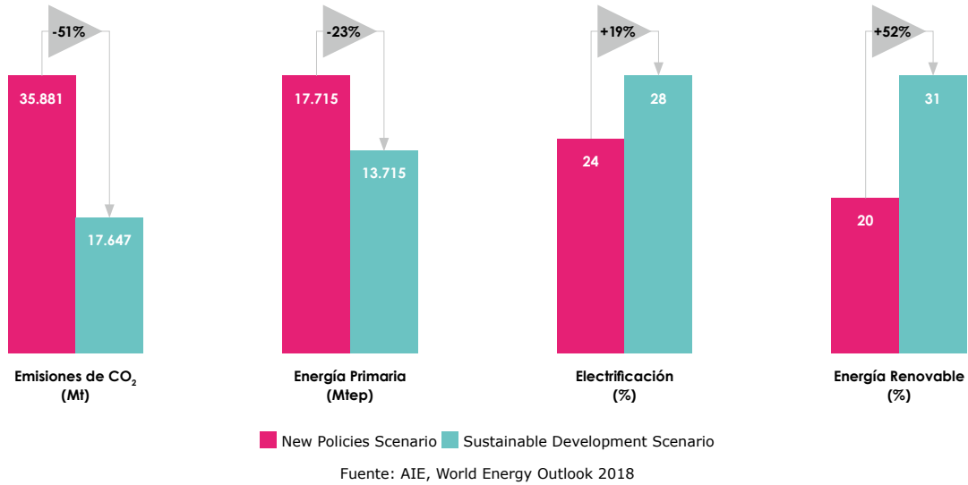
OBJETIVOS PARA CUMPLIR EL ACUERDO DE PARIS EN EL MUNDO EN 2040
