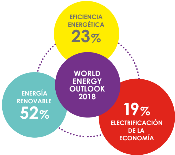
OBJETIVOS PARA CUMPLIR EL ACUERDO DE PARIS EN EL MUNDO EN 2040
